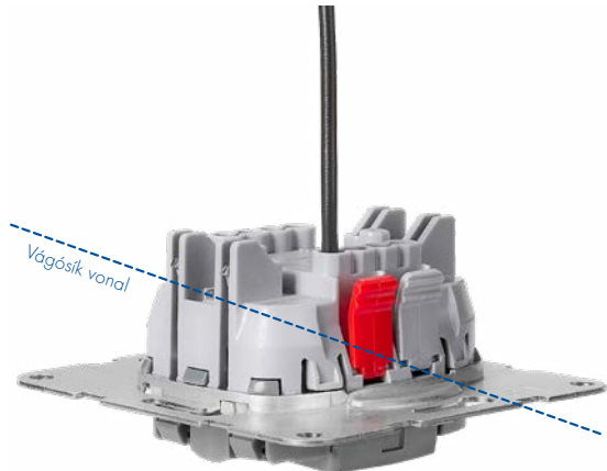
Kapcsoló keresztmetszet
