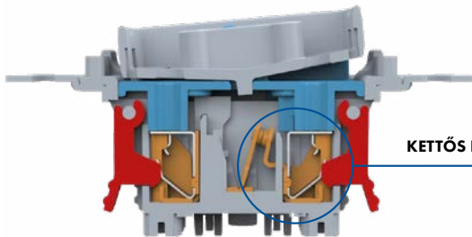
Kapcsoló keresztmetszet
