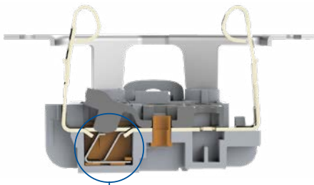
Aljzat keresztmetszet
