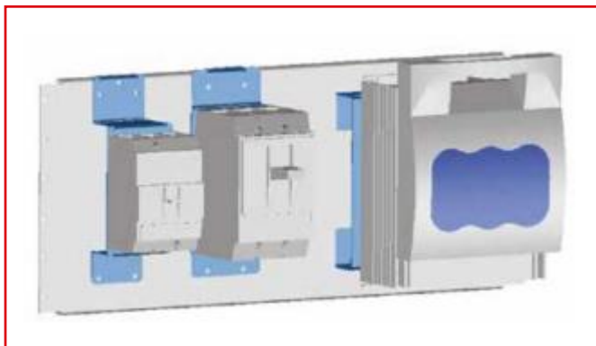
Részleges szerelőlap alkalmazási példa
