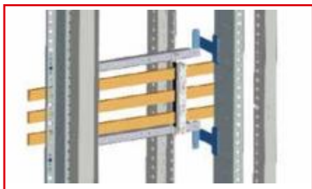
HU1L900304 használata
