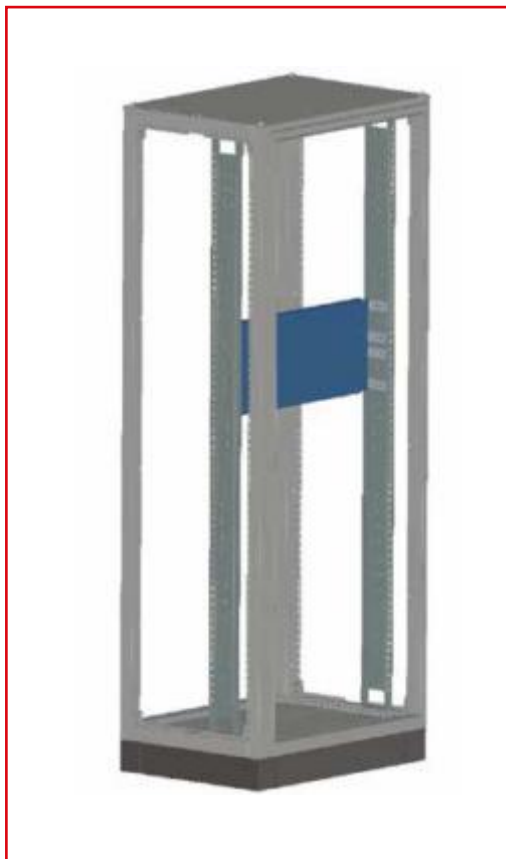
HUMIMP3008 szerelőlap elhelyezése HUMI2000 szerelőbetétben
