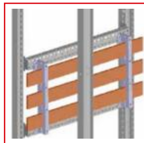
100 mm sínrendszer használata
