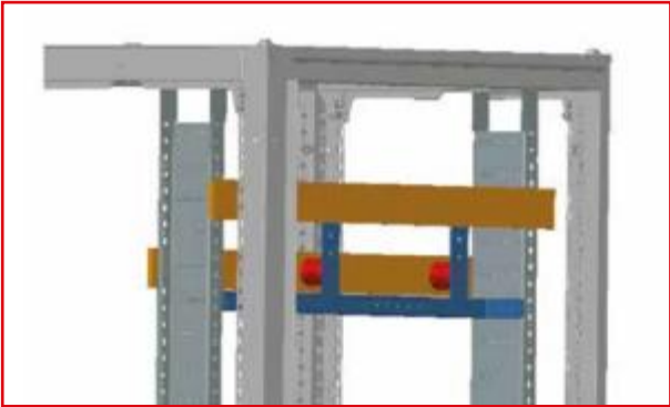
HUMINPE100 használata
