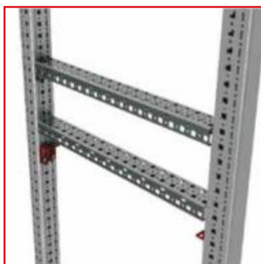
ATCLF020-- használata
